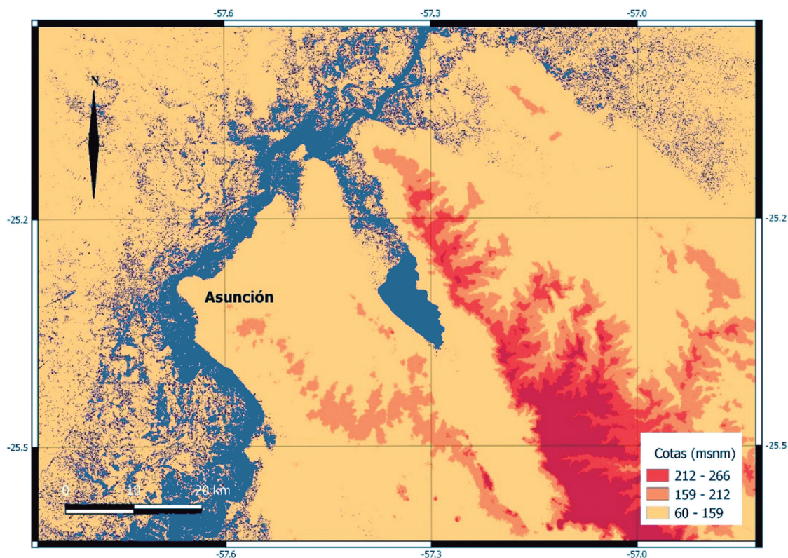
Figura 7. Regresión marina y retención de un cuerpo de agua en los mínimos topográficos del valle de Ypacarai durante el Mioceno tardío – Plioceno temprano (7.24 a 3.60 millones de años).
