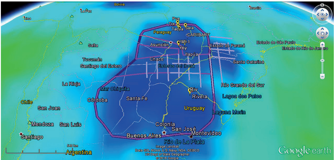
Figura 10. Corazón Archon del Cratón Río de la Plata, modelo actualizado (up-grade) en proceso de depuración a los previos presentados por Presser (2010, 2011 y 2014) basado en tomografía sísmica del modelo de TX2011 (dVs %) -comentarios en el texto. Bordes en conjunto en línea gruesa dentro de los que se trazan 2 grandes bloques Archon; al N. 1-Apa con indicación de las localidades diamantíferas comentadas en el texto; Pue-Puentesíño; Tre-Trementina; Sara-Cerro Sarambi-Cerro Chiriguelo; Tacua-Tacuati; Capiibary, Ymi-1 y Yby-Ybytyruzu. Al S. 2-Plata donde en Uruguay la localidad de diamante aluvial y lamprófidos ultramáficos es localizada próxima a la localidad de Riviera -Riv. Entre ambas un tercer pequeño bloque (visto como Archon/Protón o Archon re-trabajado) el Tebicuary. Base del mapa, tomografía sísmica en 2D a 200 km del modelo de TX2011 (dVs %) global; notar que el corazón Archon se sitúa en la zona azul (mayor velocidad). Las líneas verticales y horizontales entre-cruzadas corresponden a zonas de un potencial manto anómalo.
